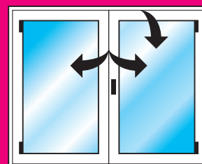
Oscillo-battant, ferrage symétrique
